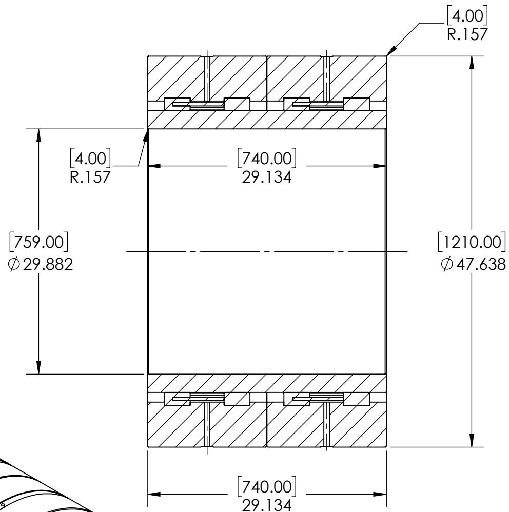
SECTION A-A
