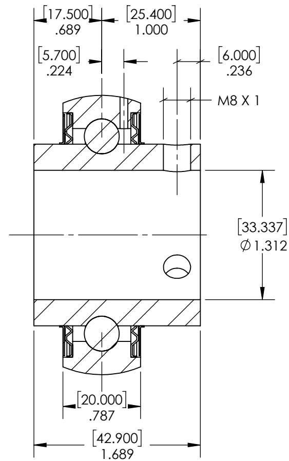
SECTION A-A
