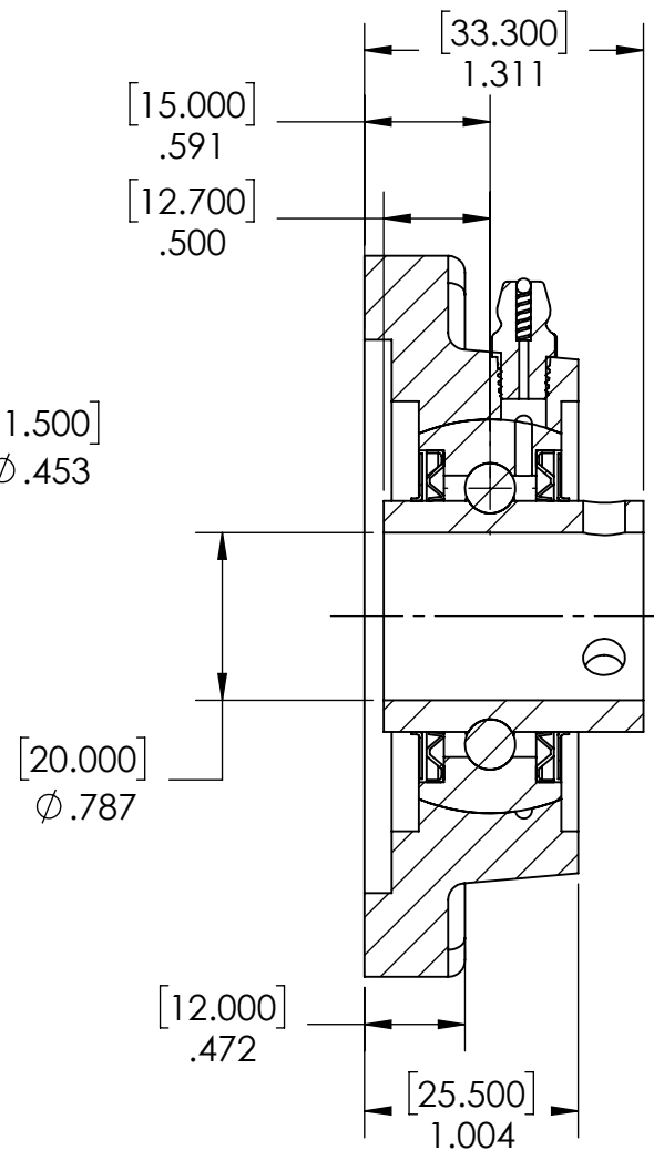
SECTION A-A
