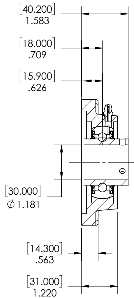
SECTION A-A
